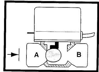
Без подачи электричества (рис. 1)
